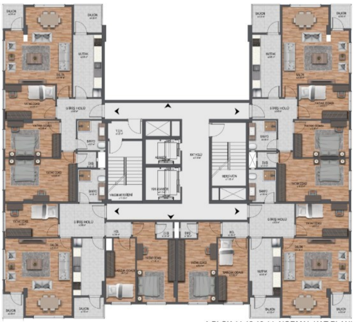
A BLOK 11.12.13.14. NORMAL KAT PLANI kat brüt alanı : 500,90 m 2 .
